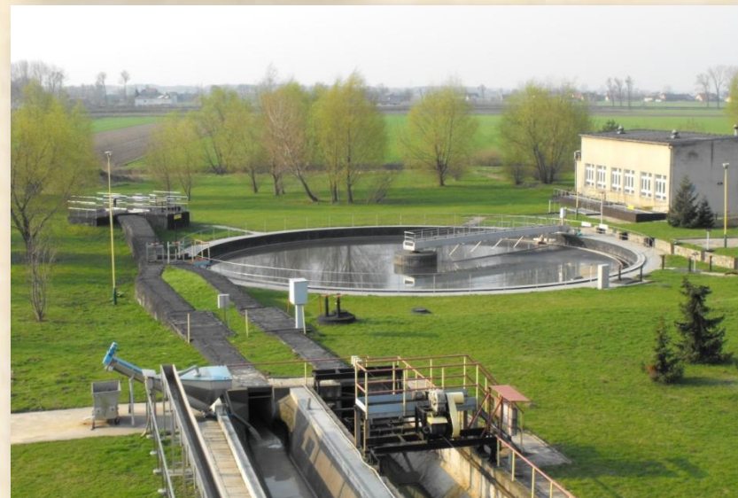
Biologiczno – mechaniczna oczyszczalnia ścieków w Krotoszynie.
